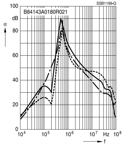
Filter für 180 A
