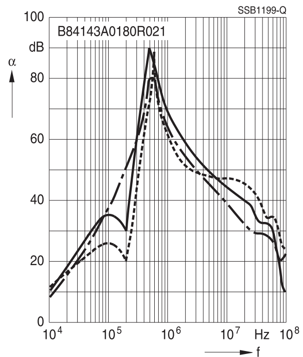
Filter für 180 A
