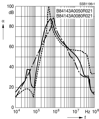
Filter für 50 A und 80 A
