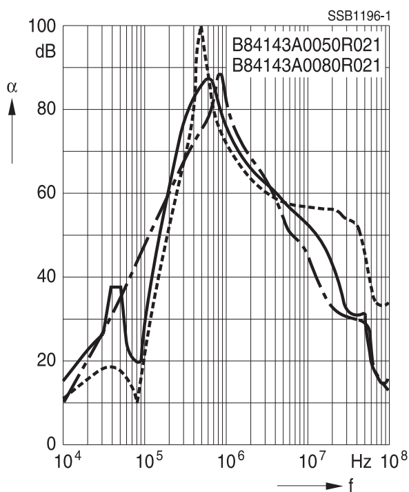
Filter für 50 A and 80 A
