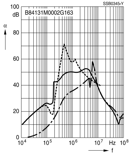
Filter für 125 A
