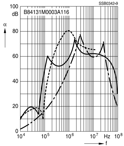
Filter für 35 A
