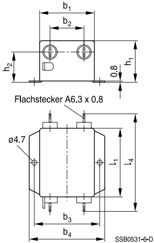
B84114D0000A010 ... A60 (1 A ... 6 A)
