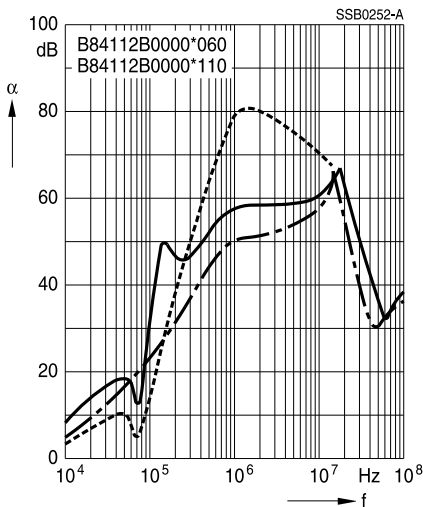
Filter für 6 A und 10 A
