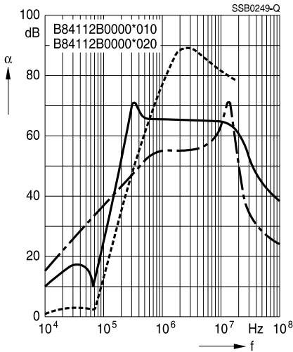
Filter für 6 A und 10 A
