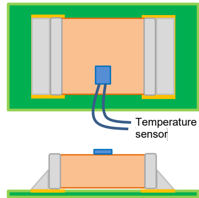
CL2220 350 V Soft termination (Z63000Z2910Z1Z56 #)
