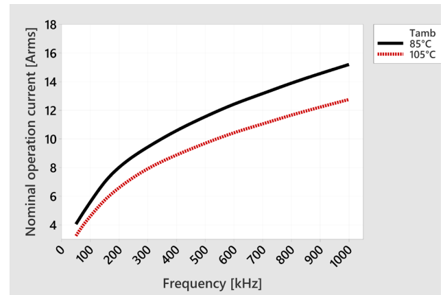
CL2220 350 V Soft termination (Z63000Z2910Z1Z56 #)
