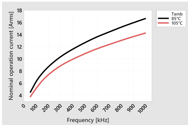
CL2220 350 V Standard termination (Z63000Z2910Z1Z54 #)
